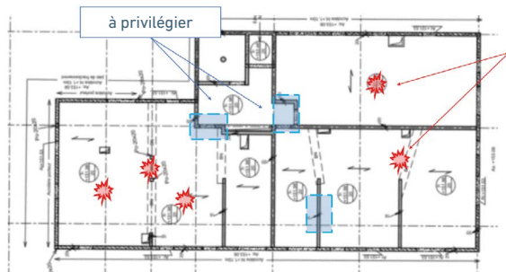
Installation de la PAC au-dessus des parties communes.
